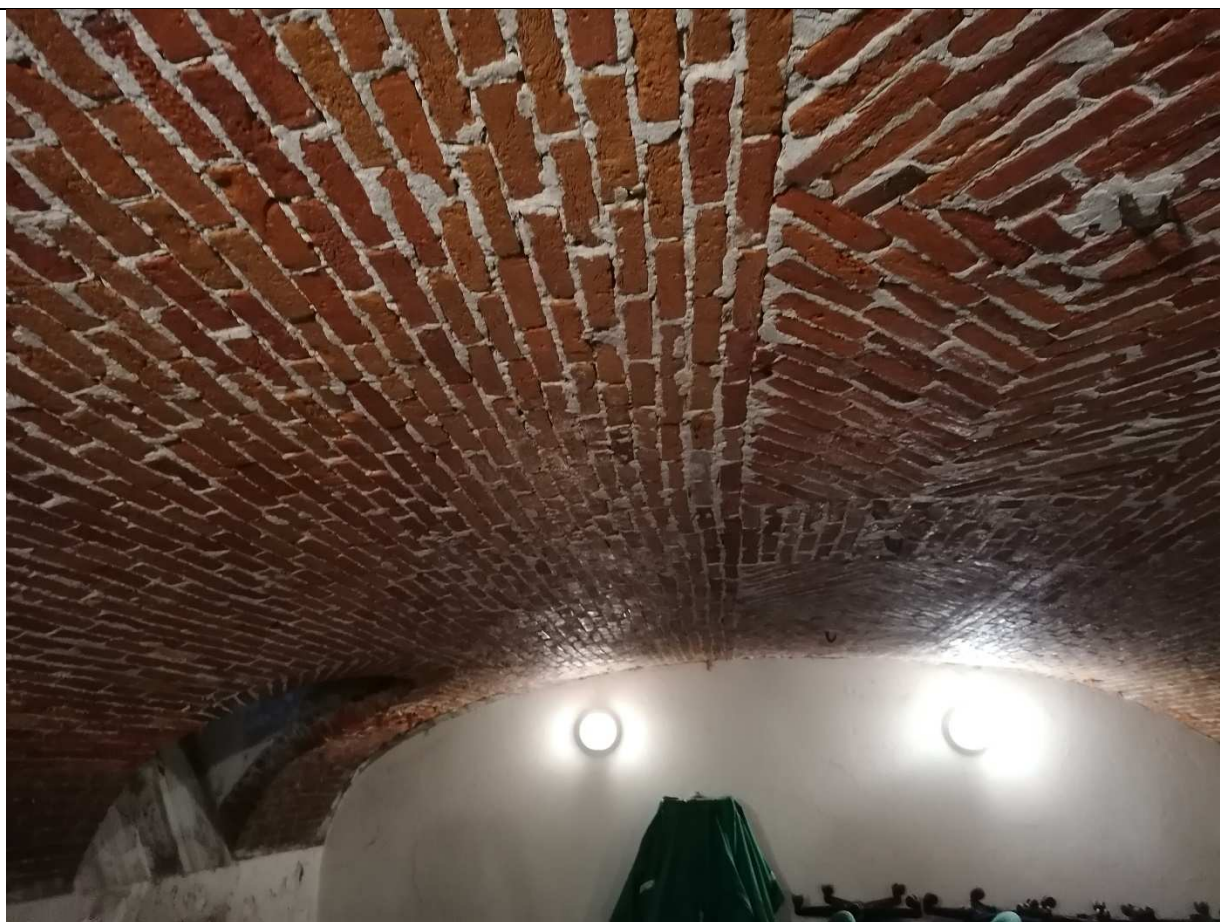
Figura 11 - locale cantina piano interrato
